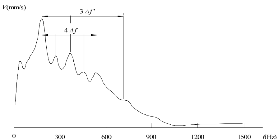
图5 缺陷桩典型速度幅频信号特征
