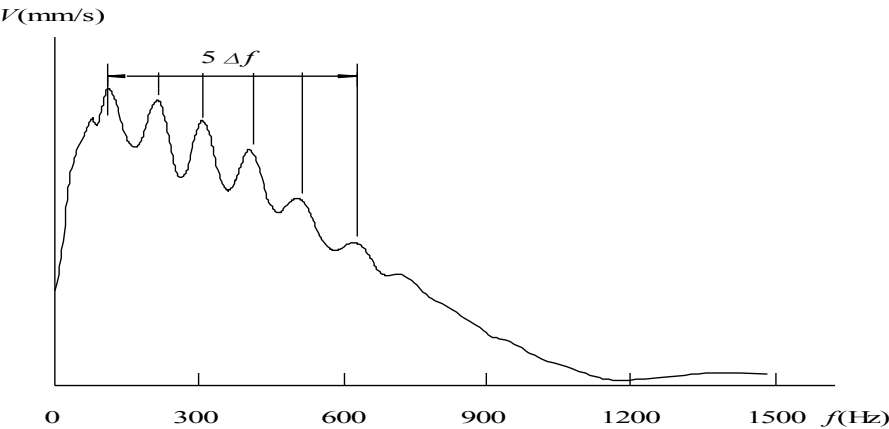
图 3 完整桩典型速度幅频信号特征
