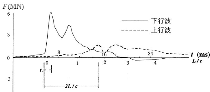
图 9.4.3 桩身波速的确定
