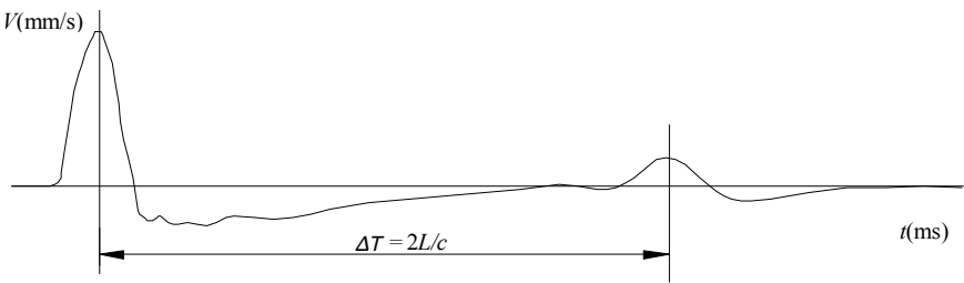
图 2 完整桩典型时域信号特征
