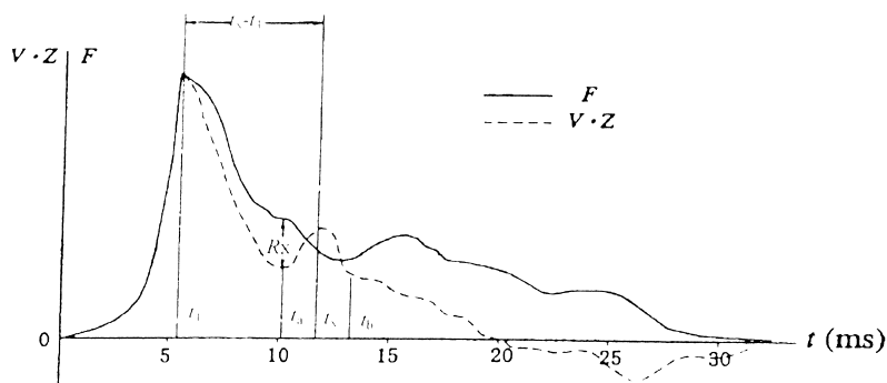
图 9.4.12 桩身完整性系数计算
