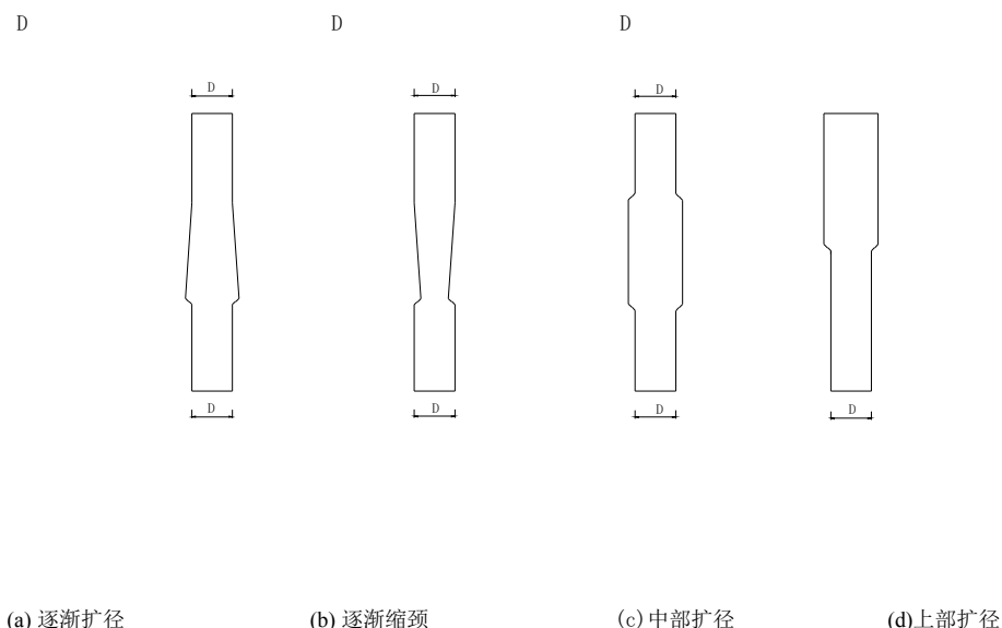
图 7 混凝土灌注桩截面(阻抗)变化示意图
